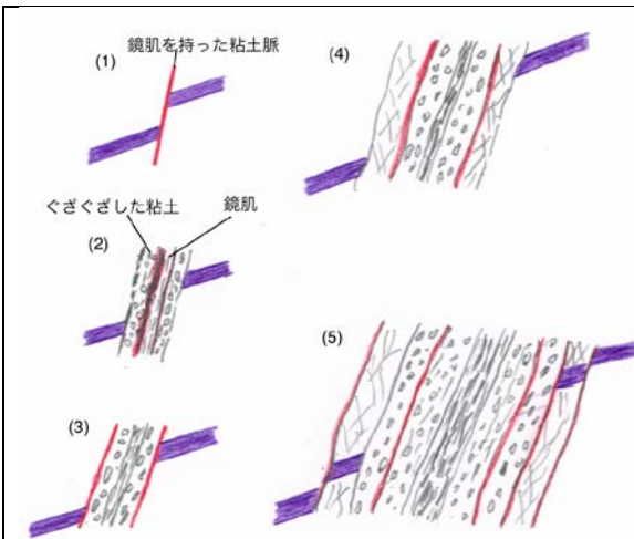
【図 5.6 丹那トンネルでの断層のいろいろ（鐵道省熱海建設事務所，1933，丹那トンネルの話〈復刻版〉，173pより）】
