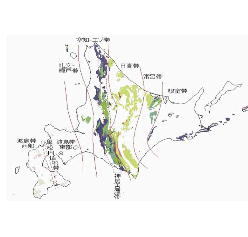
【図 5.4 北海道の中生界・古生界の地質構造】
